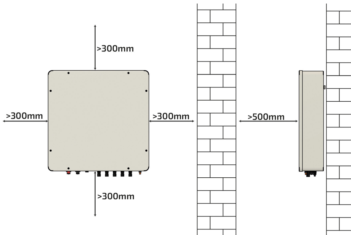
Abbildung 25. Montagebedingungen — Parallelschaltbox
