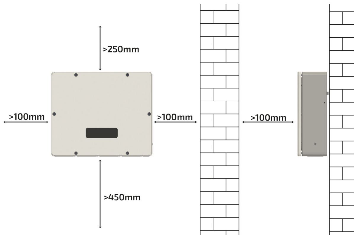
Abbildung 26. Montagebedingungen – STS-Box
